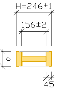
Lõige A-A
