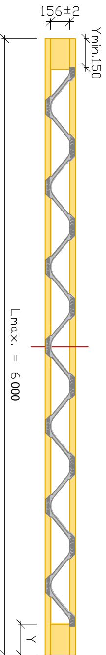
Lõige A-A
